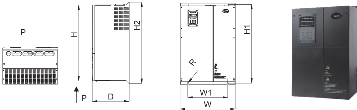
SM10/22系列外型及安装尺寸示意图
