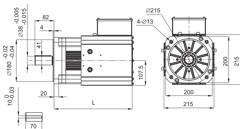
200机座安装尺寸示意图
